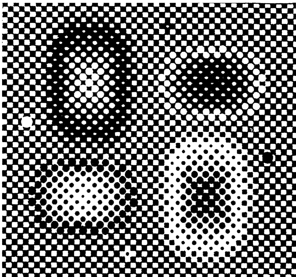
الشكل ٧ - المجرات
